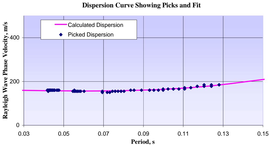
Figura 2: Diagramma periodo – velocità di fase tratto dalla prova Re.Mi.
