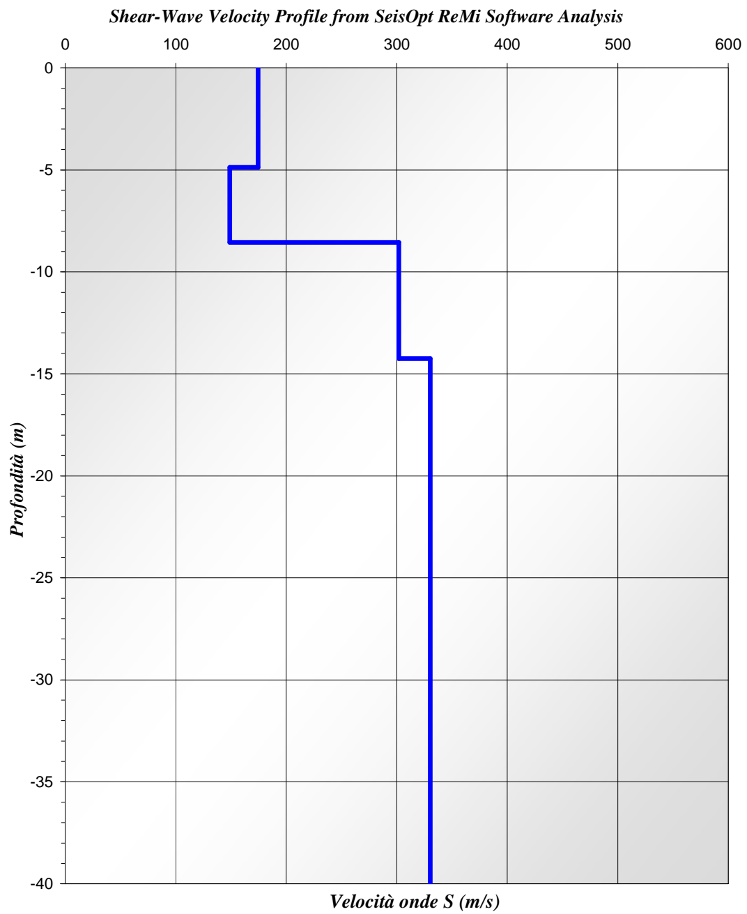
Figura 3: modello interpretativo, tratto dalla prova Re.Mi., le cui modifiche influenzano direttamente la curva di dispersione.
