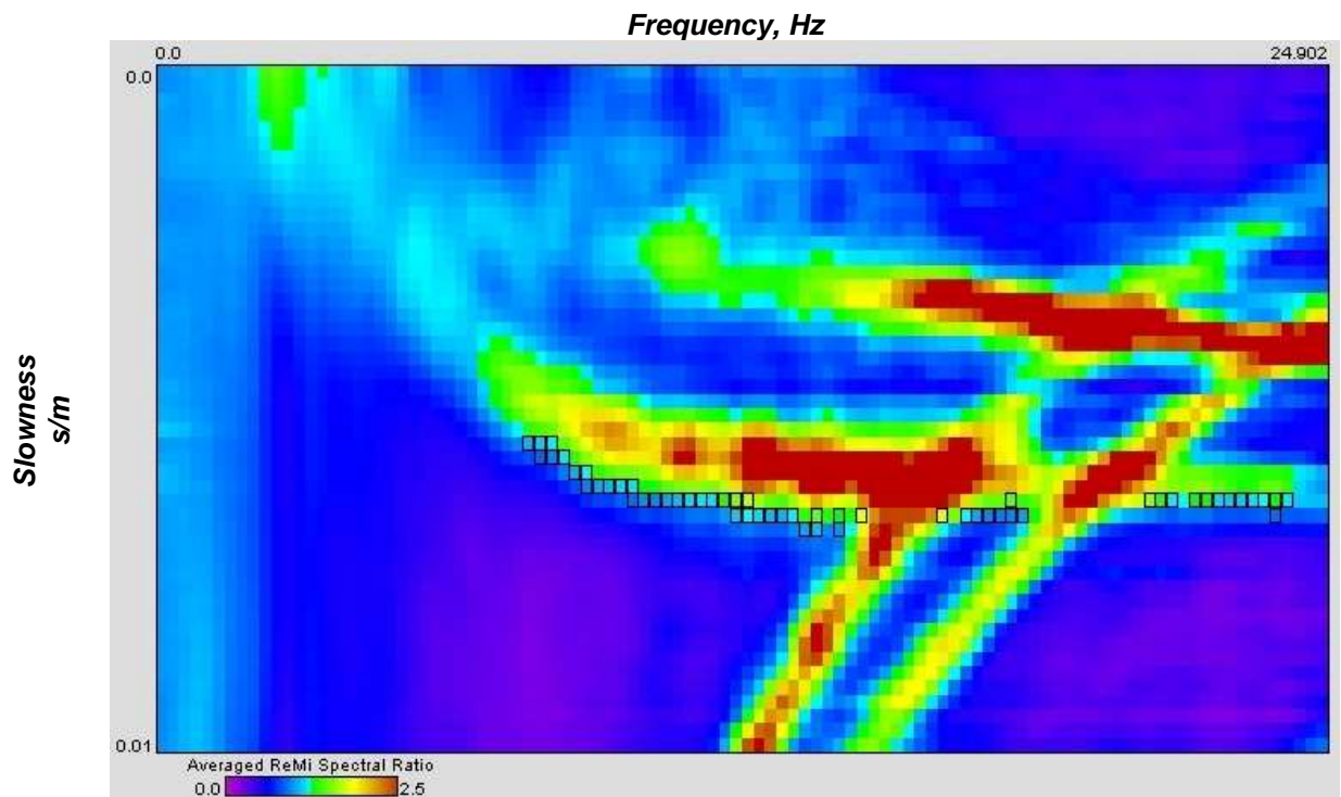
Figura 1: grafico p-f tratto dalla prova Re.Mi.
